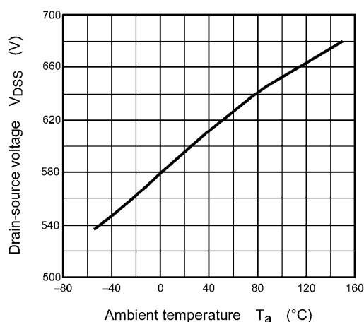
Fig. 8.5 V_{DS} - T_a
