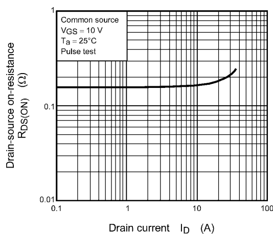
Fig. 8.6 R_{DS(ON)} - I_D
