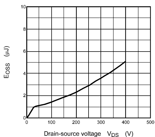
Fig. 8.10 E_{OSS} - V_{DS}
