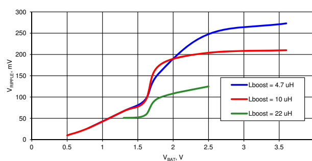
Figure 11-14. V_{RIPPLE} vs V_{BAT} [28]
