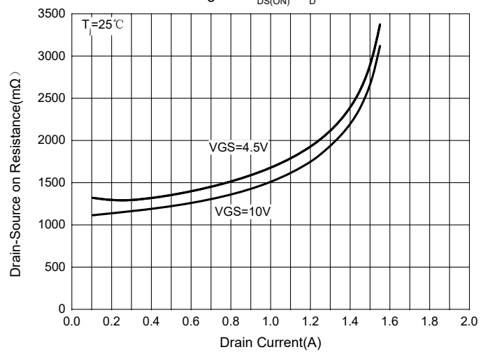
Fig. 3 - R_{DS(ON)} - I_D
