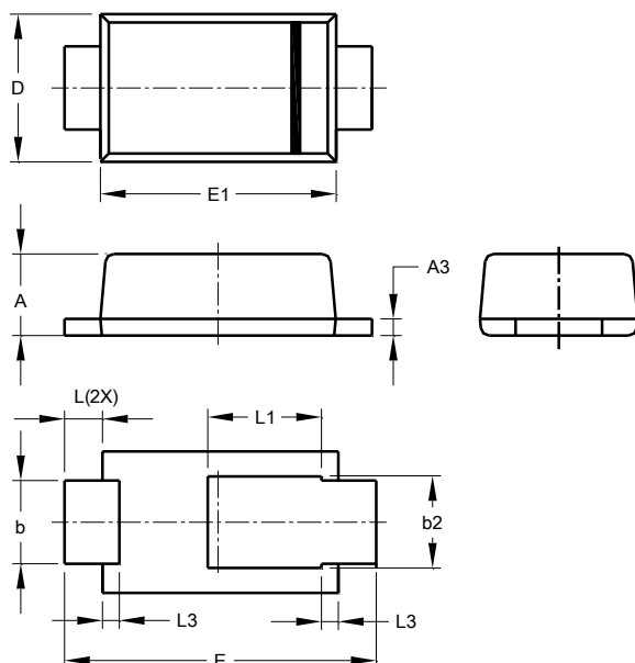
PowerDI123
