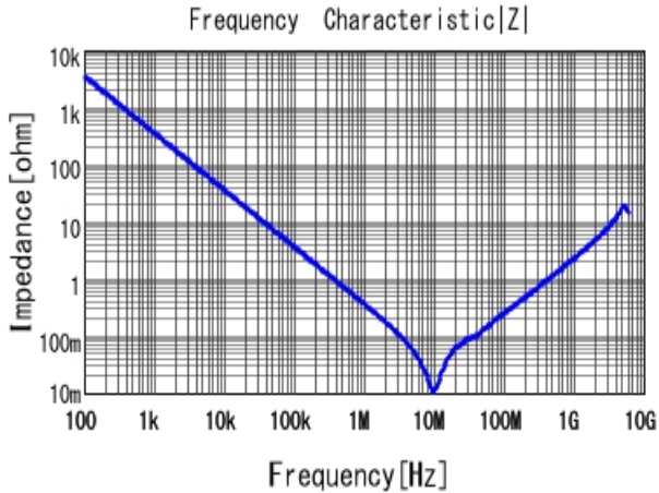
■ GCM219R71E474KA55 |Z| DC0V, 25degC
