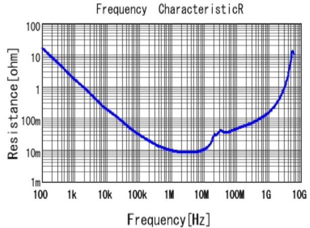
■ GCM219R71E474KA55 R DC0V, 25degC
