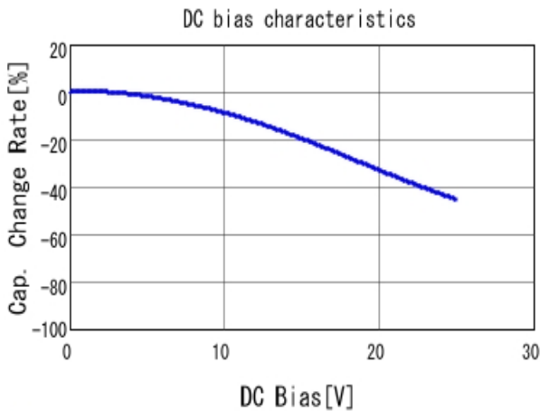
■ GCM219R71E474KA55 C-DC bias capchange, 25.0degC, AC1.
