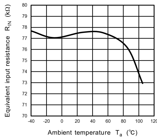
Fig. 12.10 R_{IN} - T_a
