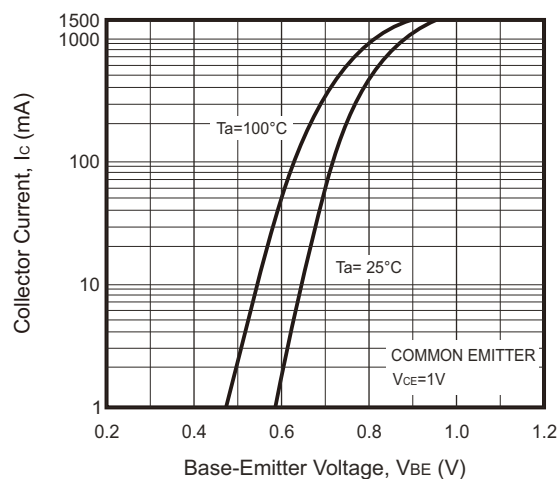
Fig.5 - V_{BE} - I_c
