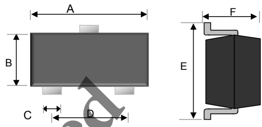
SOT-323
