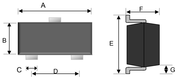
SOT-23
