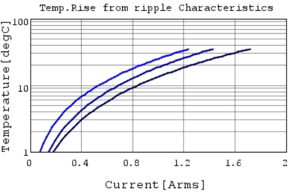
GRM155C8YA224KE01 Temp.rise 300kHz
