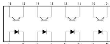
TLP621-4
