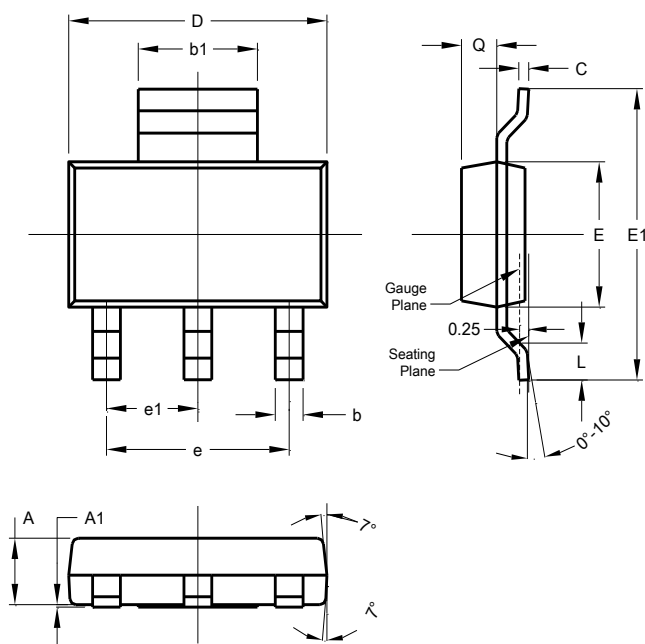
SOT223
