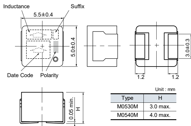
PCC-M0530M type PCC-M0540M type (ETQP3M□□□YFP/ETQP4M□□□YFP)
