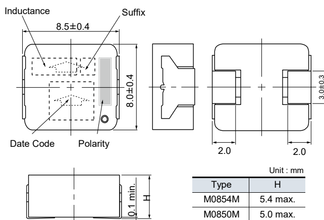
PCC-M0854M type PCC-M0850M type (ETQP5M□□□YFK/GAK/YGK)
