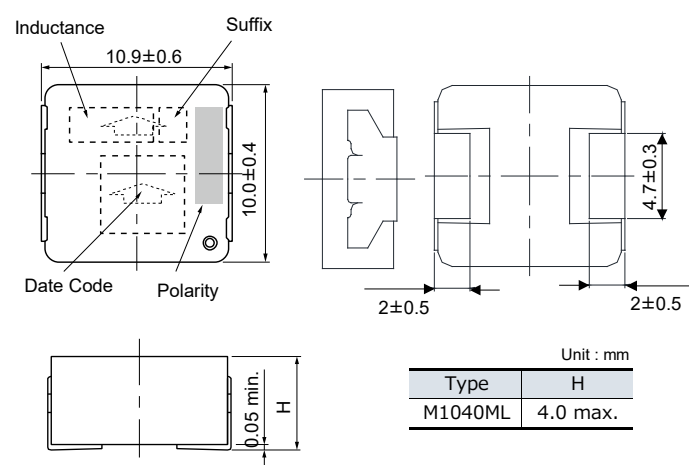
PCC-M1040ML type (ETQP4M□□□KLC)
