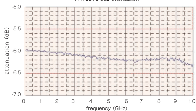
PAT0816 6dB attenuation
