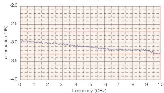
PAT0816 3dB attenuation
