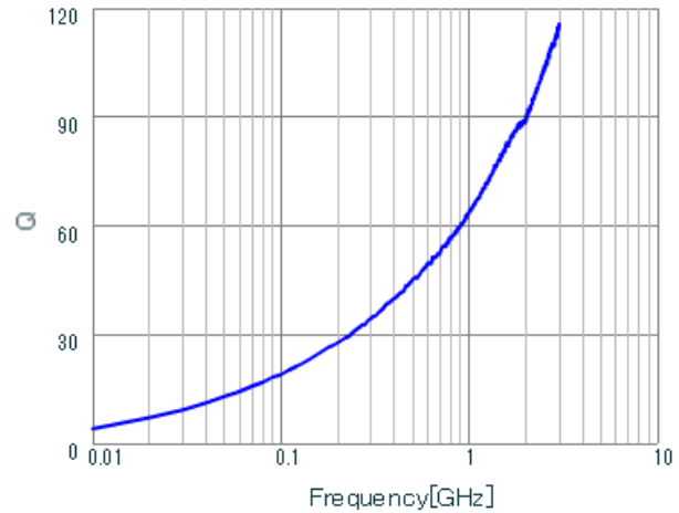
LQW15AN3N9D00 Q.
