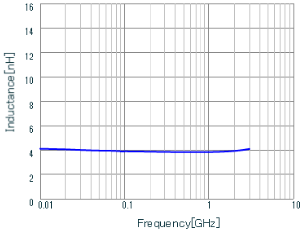
LQW15AN3N9D00 L.
