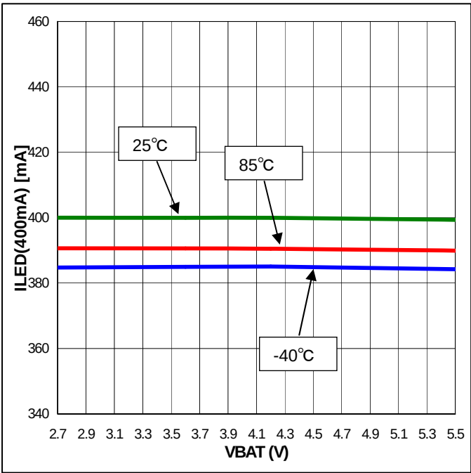
Figure 5-4. ILED(400mA) - VBAT
