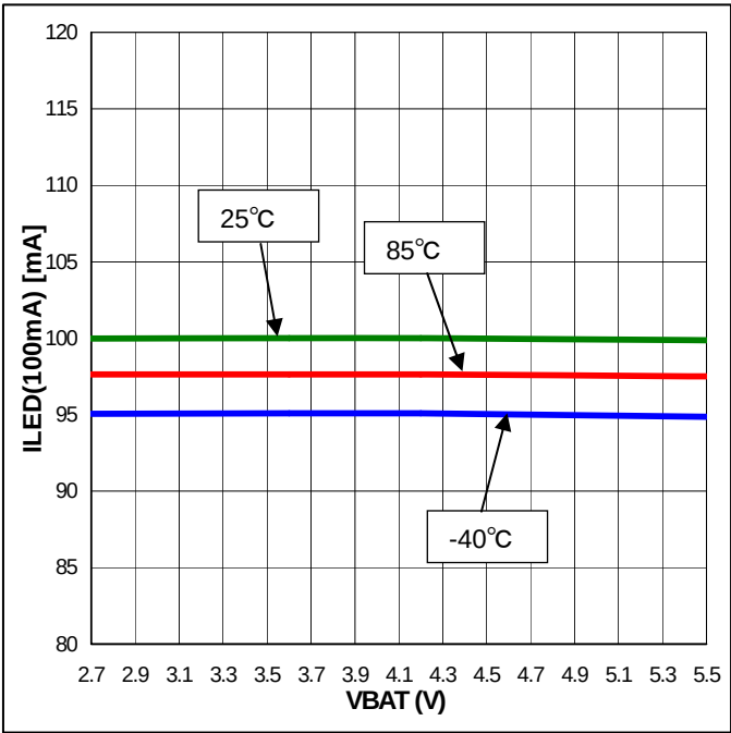
Figure 5-3. ILED(100mA) – VBAT
