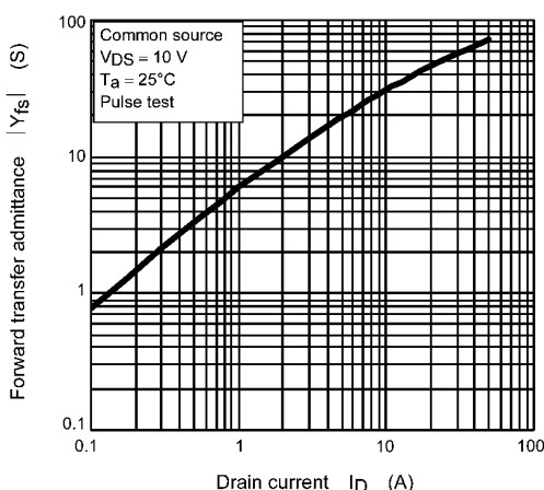
Fig. 8.5 |Y_{fs}| - I_D
