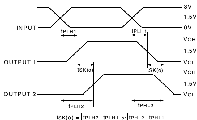
Output Skew
