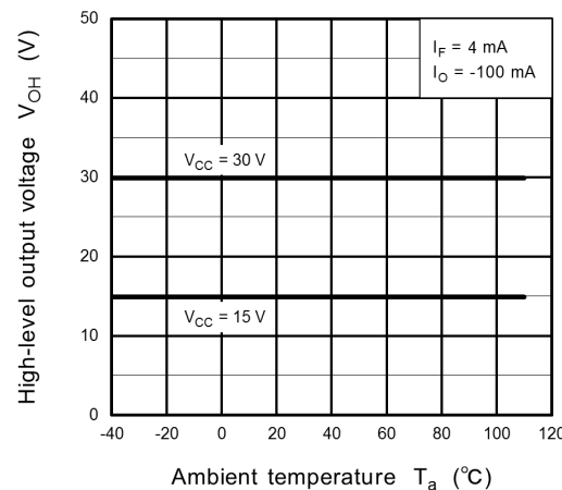
Fig. 13.2.8 V_{OH} - T_a
