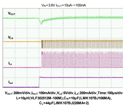
XC9265A301
