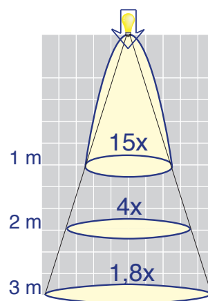
PL121106 (13°) - 3 METER
