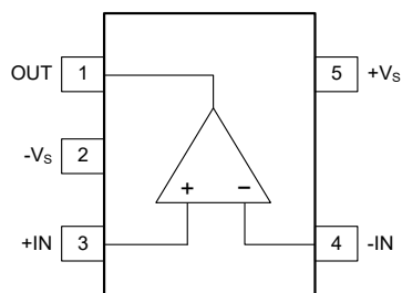
SOT-23-5
