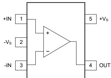
SOT-23-5
