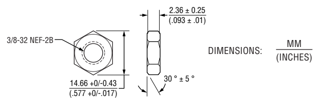
NUT H-38-2
