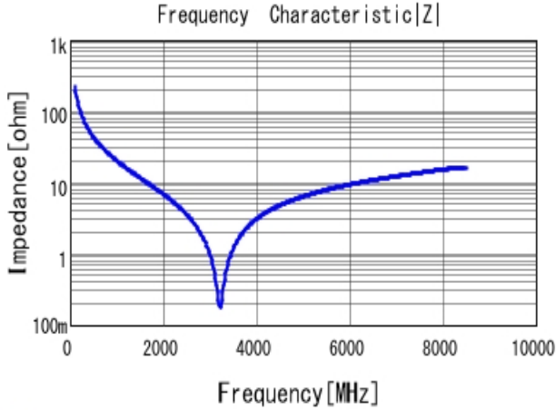
■ GCQ1555C1H7R1CB01 |Z| DC0V, 25degC
