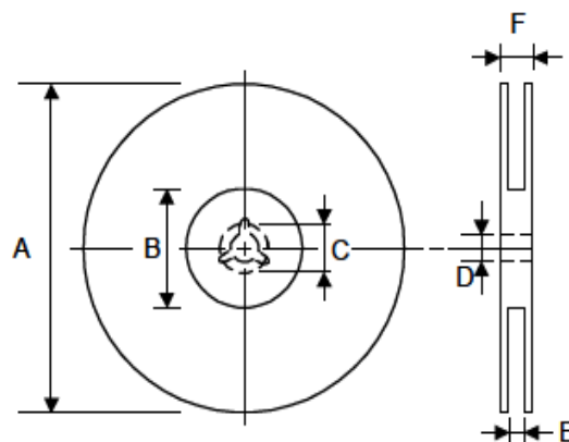
Reel Dimensions
