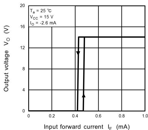
Fig. 12.2.13 V_O - I_F
