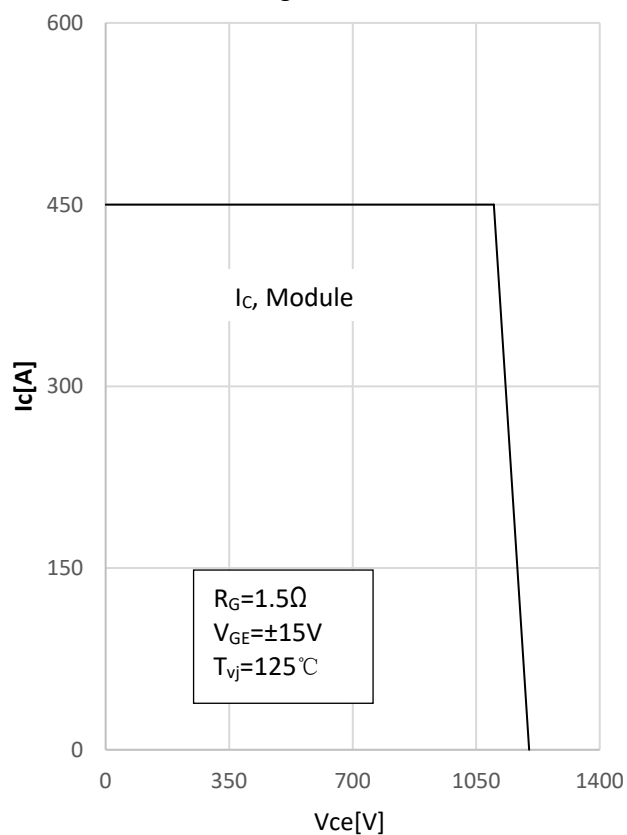
Fig5.RBSOA
