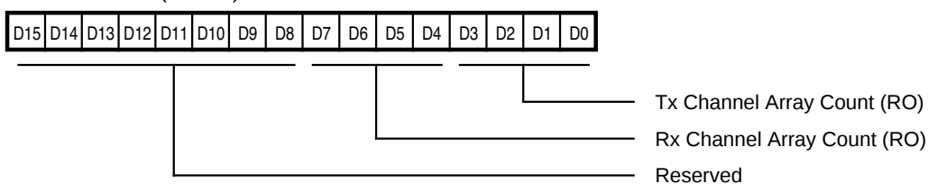
Figure 14a. DMA Array Count Register (DACR)
