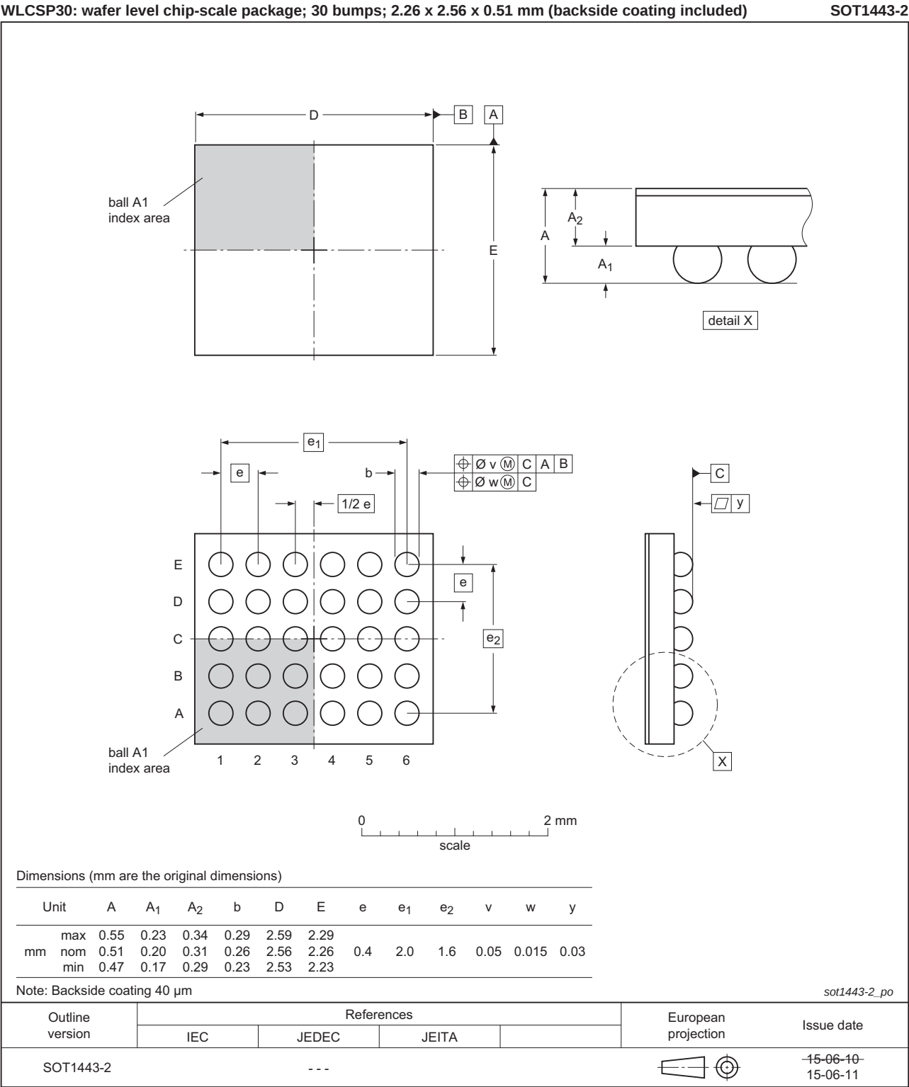
Fig 25. Package outline SOT1443-2 (WLCSP30)
