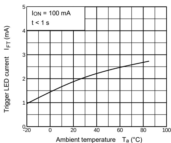
Fig.12.6 I_{FT} - T_a
