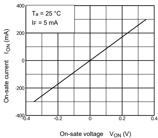
Fig.12.4 I_{ON} - V_{ON}
