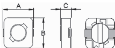
NPIS62H, NPIS64H
