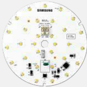
120mm / 220V
