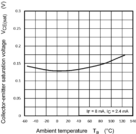
Fig. 11.13 V_{CE(sat)} - T_a
