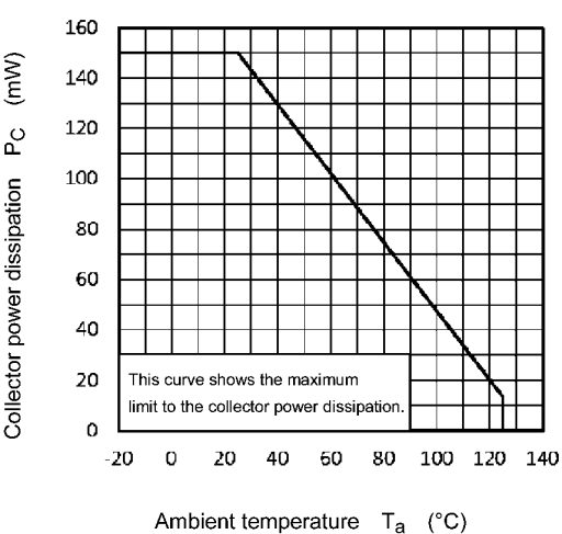
Fig. 11.2 P_C - T_a
