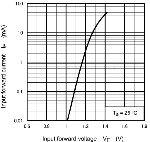
Fig. 11.4 I_F - V_F
