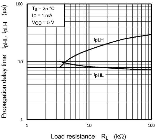
Fig. 11.14 t_{pHL}, t_{pLH} - R_L
