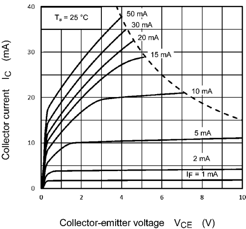
Fig. 11.7 I_C - V_{CE}
