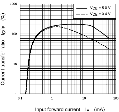
Fig. 11.11 I_C/I_F - I_F
