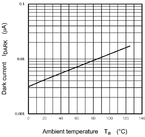
Fig. 11.10 I_{DARK} - T_a
