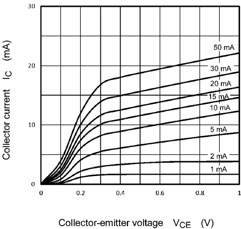
Fig. 11.8 I_C - V_{CE}
