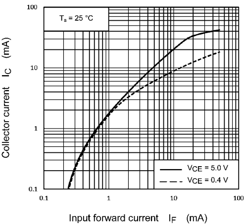
Fig. 11.9 I_C - I_F
