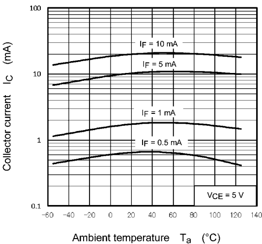
Fig. 11.12 I_C - T_a
