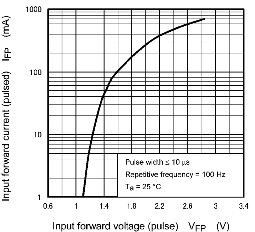
Fig. 11.6 I_{FP} - V_{FP}
