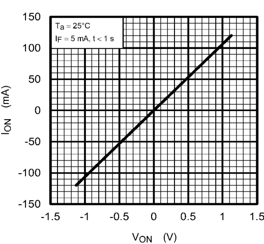
Fig. 12.4 I_{ON} - V_{ON}
