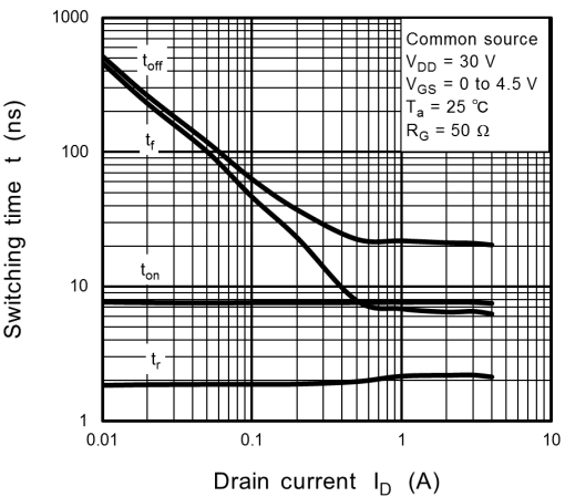
Fig. 7.9 t - I_D
