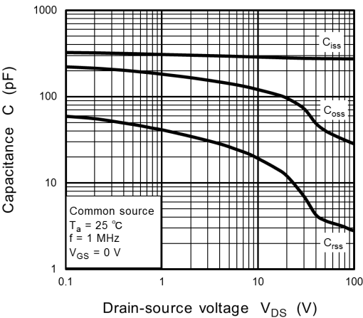
Fig. 7.7 C - V_{DS}
