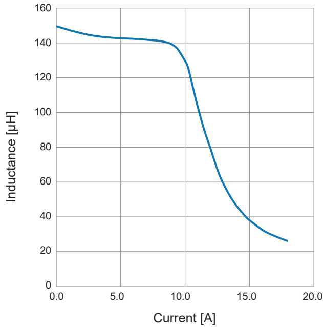
SPFC-RM12-200
