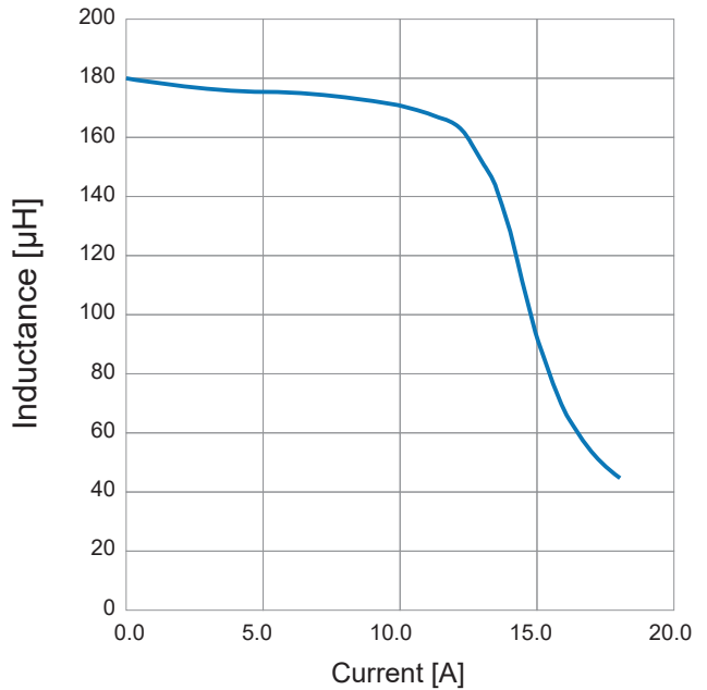
SPFC-RM14-250
