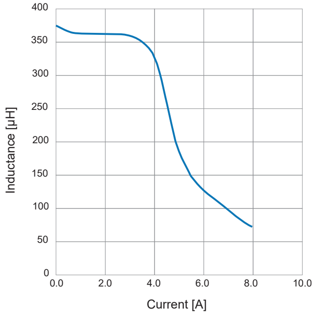
SPFC-EFD30-100
