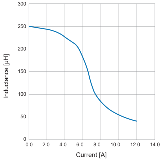
SPFC-RM10-200
