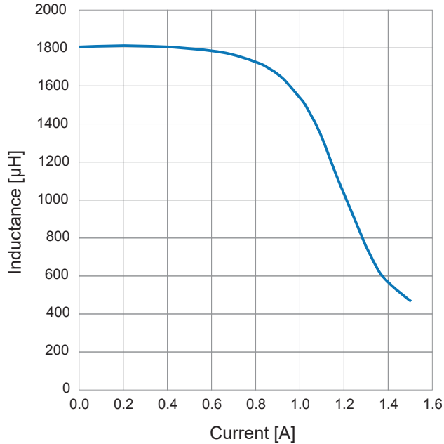
SPFC-EE20-25
