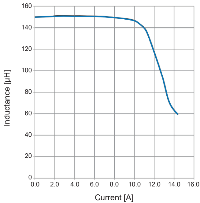
SPFC-EER28-125
