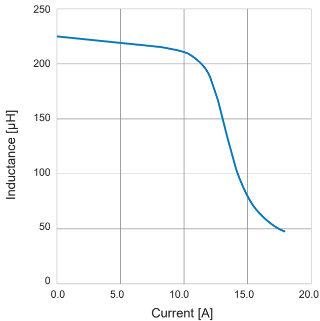
SPFC-RM14-200
