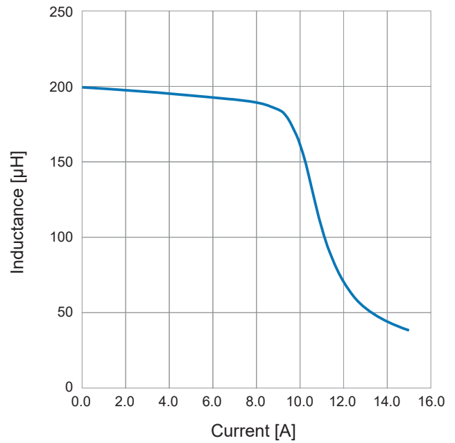
SPFC-RM12-250
