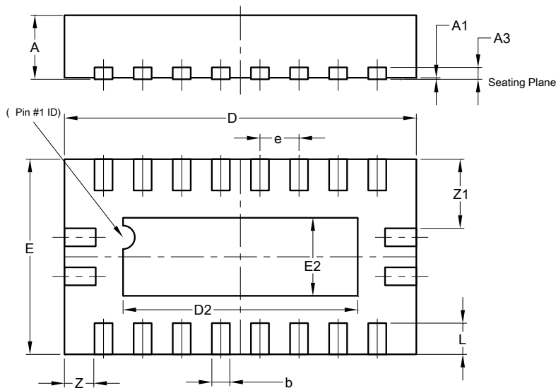
V-QFN4525-20
