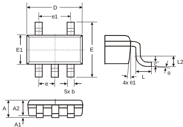
TSOT25
