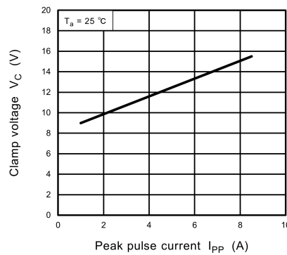
Fig. 10.6.2 V_C - I_{PP}
