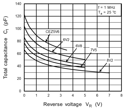
Fig. 10.1.5 C_t - V_R (1)
