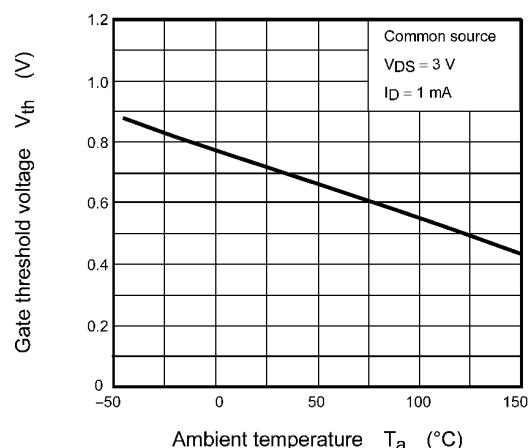
Fig. 7.6 V_{th} - T_a
