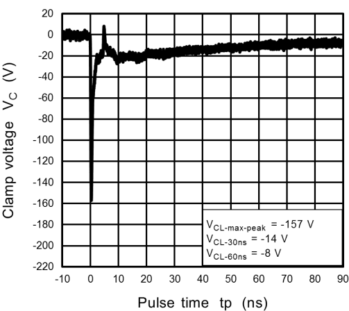
Fig. 6.1.2 -8 kV
