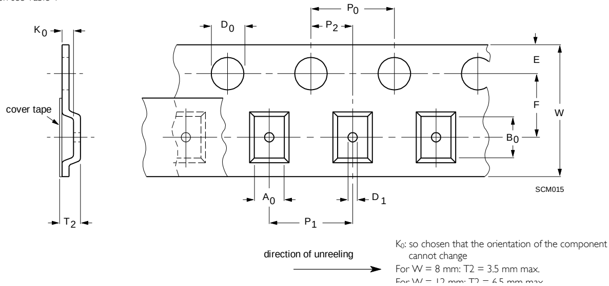
Fig. 4 Blister tape
