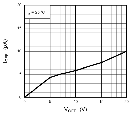
Fig. 12.9 I_{OFF} - V_{OFF}
