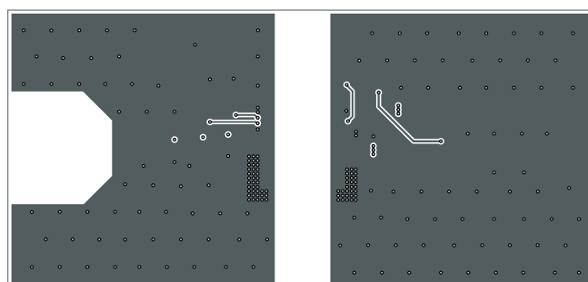
Bottom Layer
