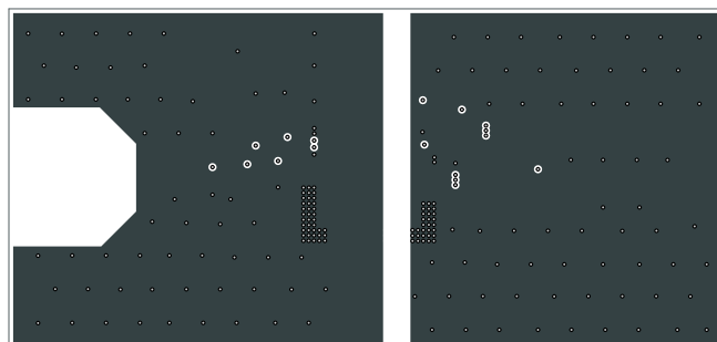
Inner Layer 1
