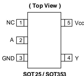
SOT25 / SOT353
