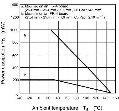
Fig. 9.14 P_D - T_a
