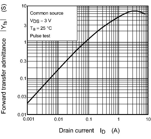
Fig. 9.8 |Y_{fs}| - I_D
