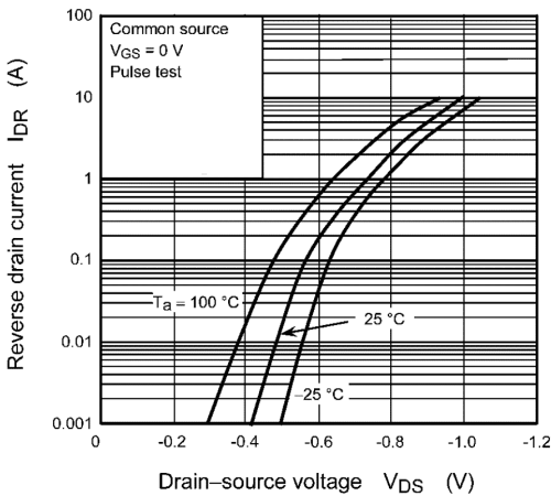
Fig. 9.9 I_{DR} - V_{DS}
