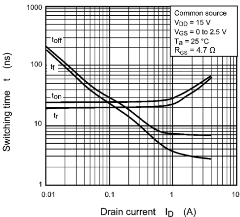
Fig. 9.11 t - I_D
