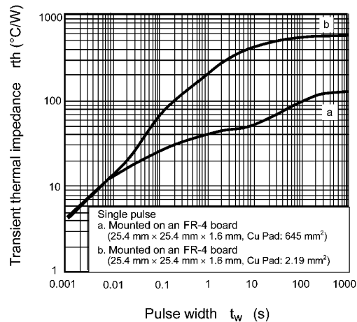
Fig. 9.13 r_{th} - t_w
