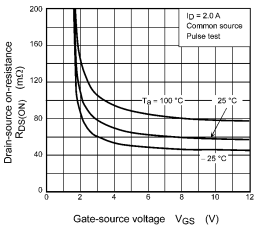
Fig. 9.4 R_{DS(ON)} - V_{GS}
