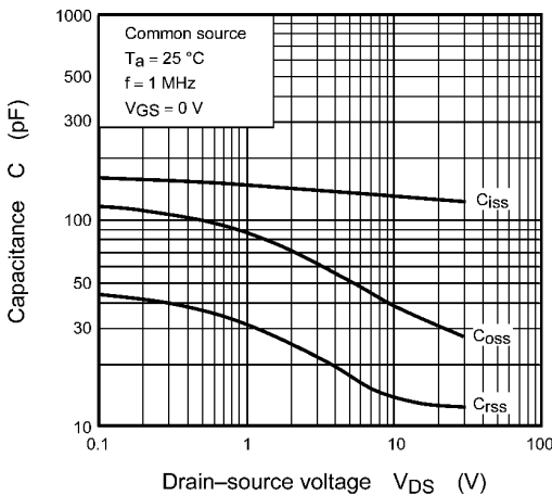
Fig. 9.10 C - V_{DS}
