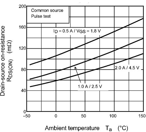
Fig. 9.6 R_{DS(ON)} - T_a
