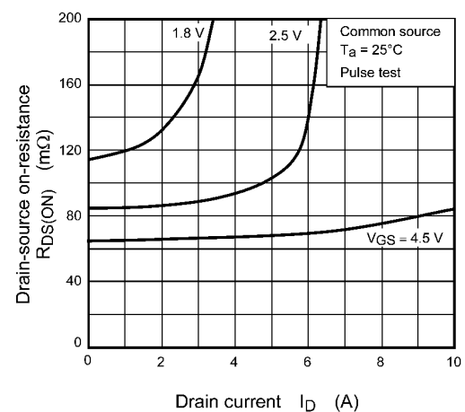
Fig. 9.5 R_{DS(ON)} - I_D
