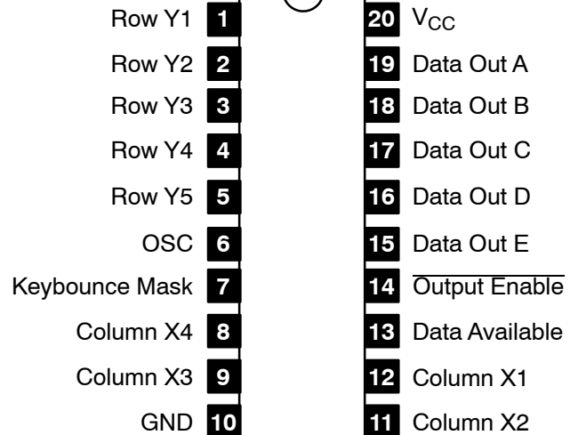
NTE74C922
