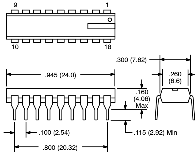
NTE74C922
