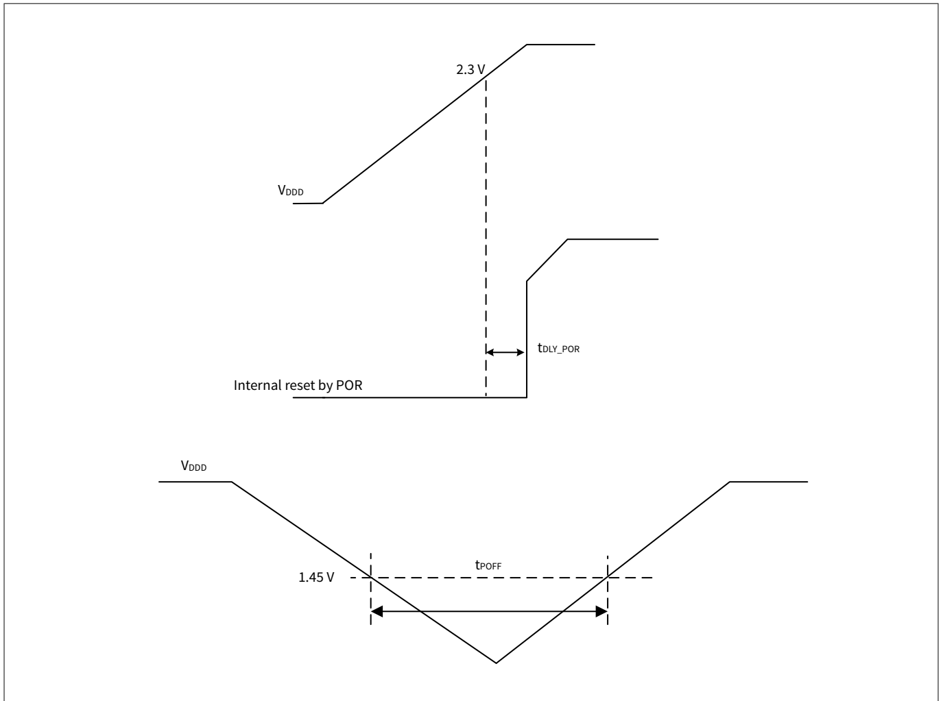
Figure 29 POR specifications
