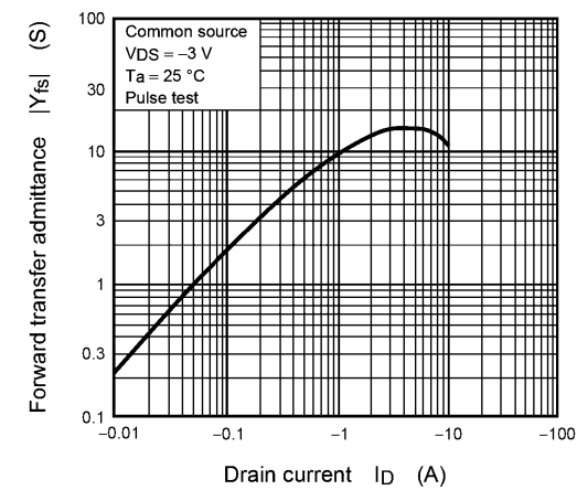
Fig. 8.8 |Y_{fs}| - I_D
