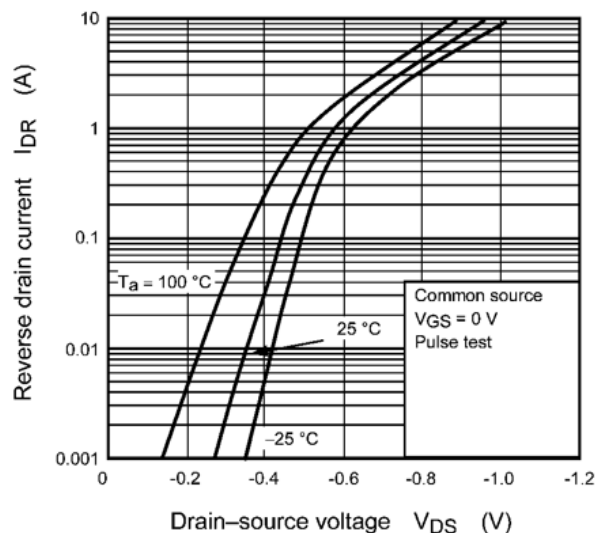
Fig. 7.9 I_{DR} - V_{DS}
