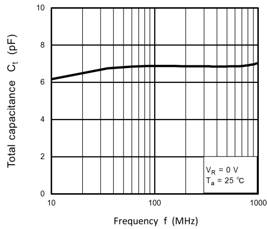
Fig. 9.4 C_t - f
