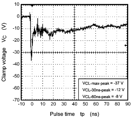
Fig. 6.1.2 -8 kV
